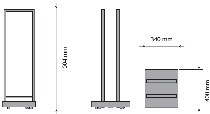
CARRITO PORTA-TRONCOS
